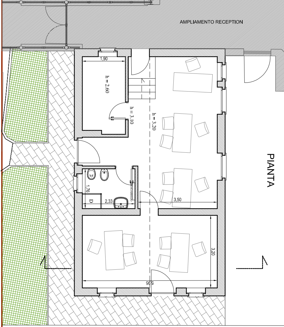
EDIFICIO 3 - STATO DI PROGETTO
