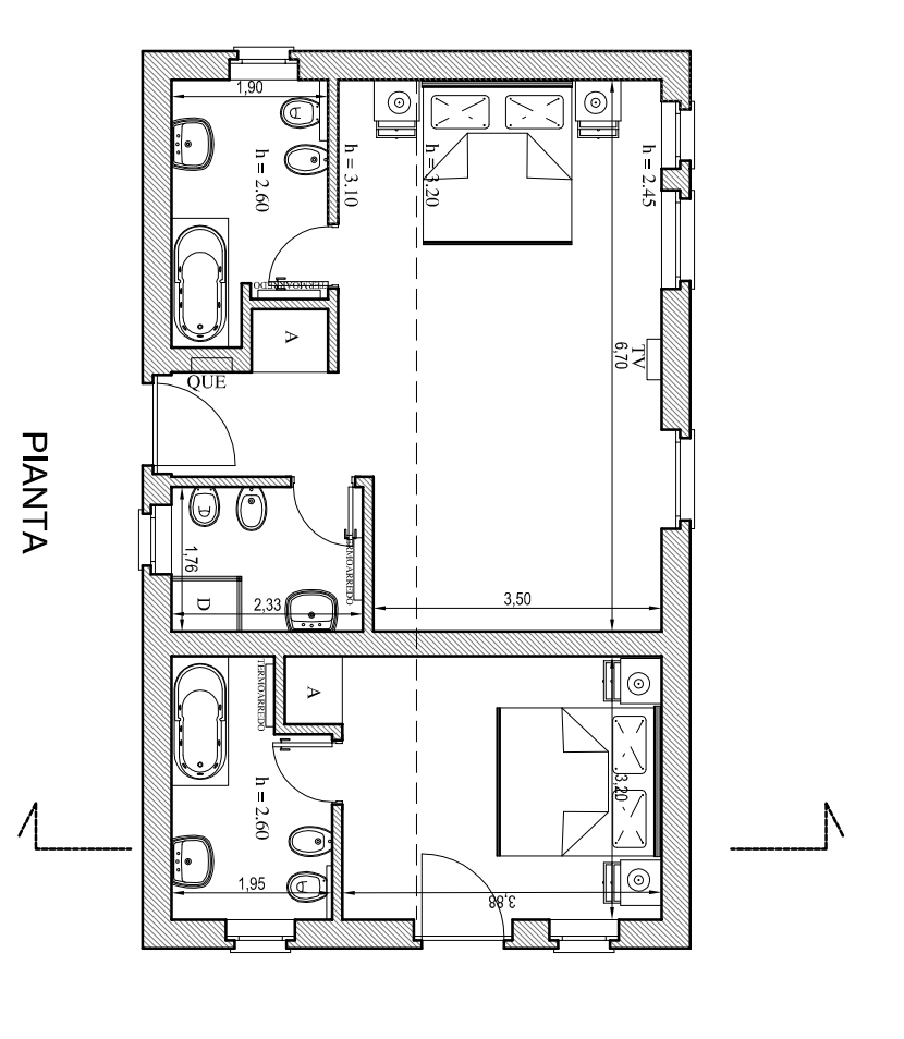
EDIFICIO 3 - STATO ATTUALE
