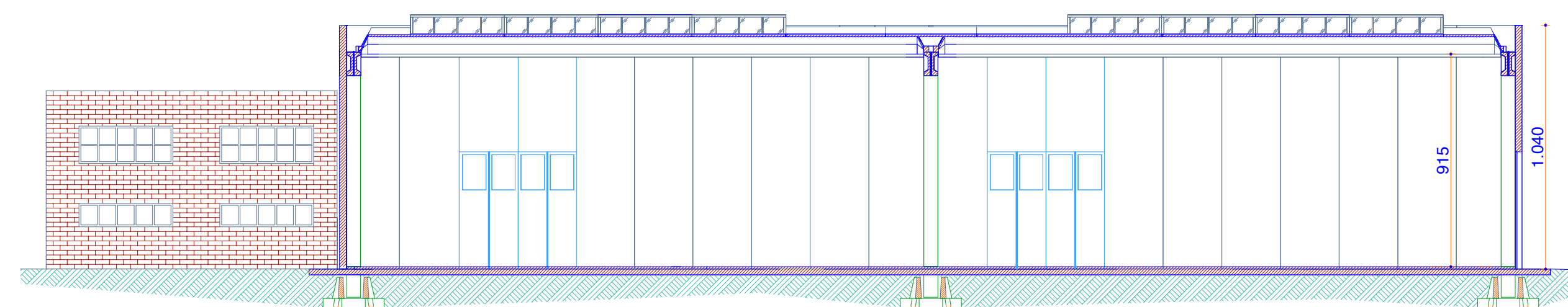
SEZIONE C - C
